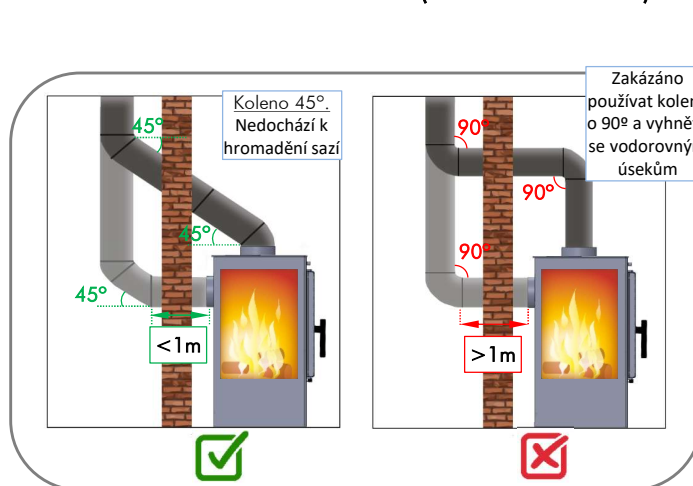
5°.- Horizontální kouřovod (hromadění sazí)
