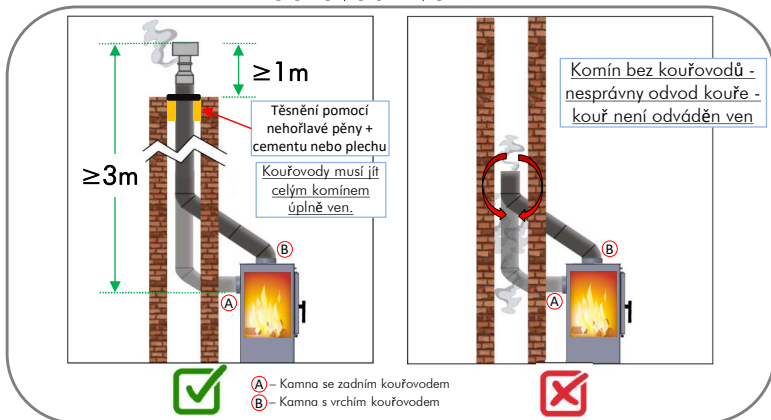
4°.- Montáž do zděného komína, odvod kouřovodů ven.
