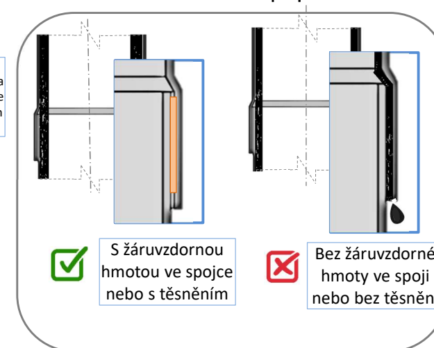
8°.- Instalace v komunitních systémech
